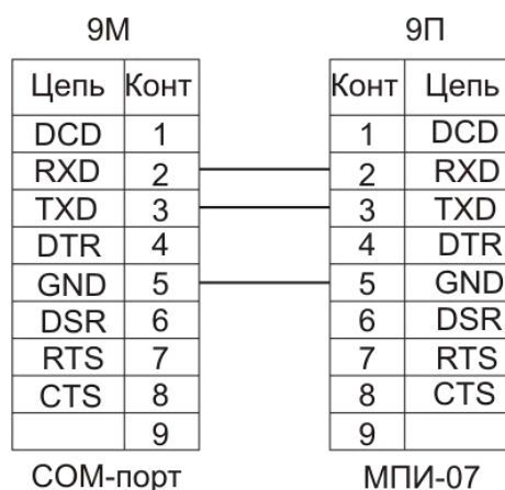
Рисунок В.1 – Схема подключения МПИ-07 к COM-порту
